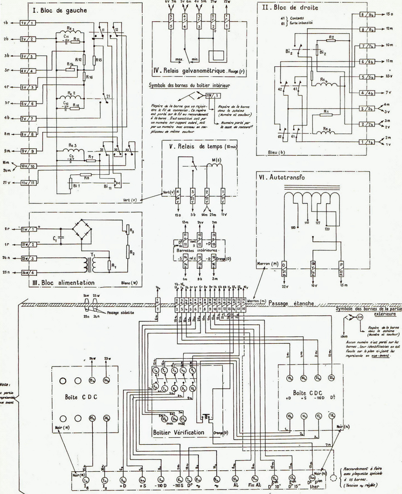
Fig. 4 — Schéma de câblage — D'après le plan : A. Le Boeuf N° 40.014
